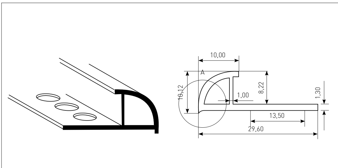
PVC Profil unutarnji UL 8 mm d=2700 mm
